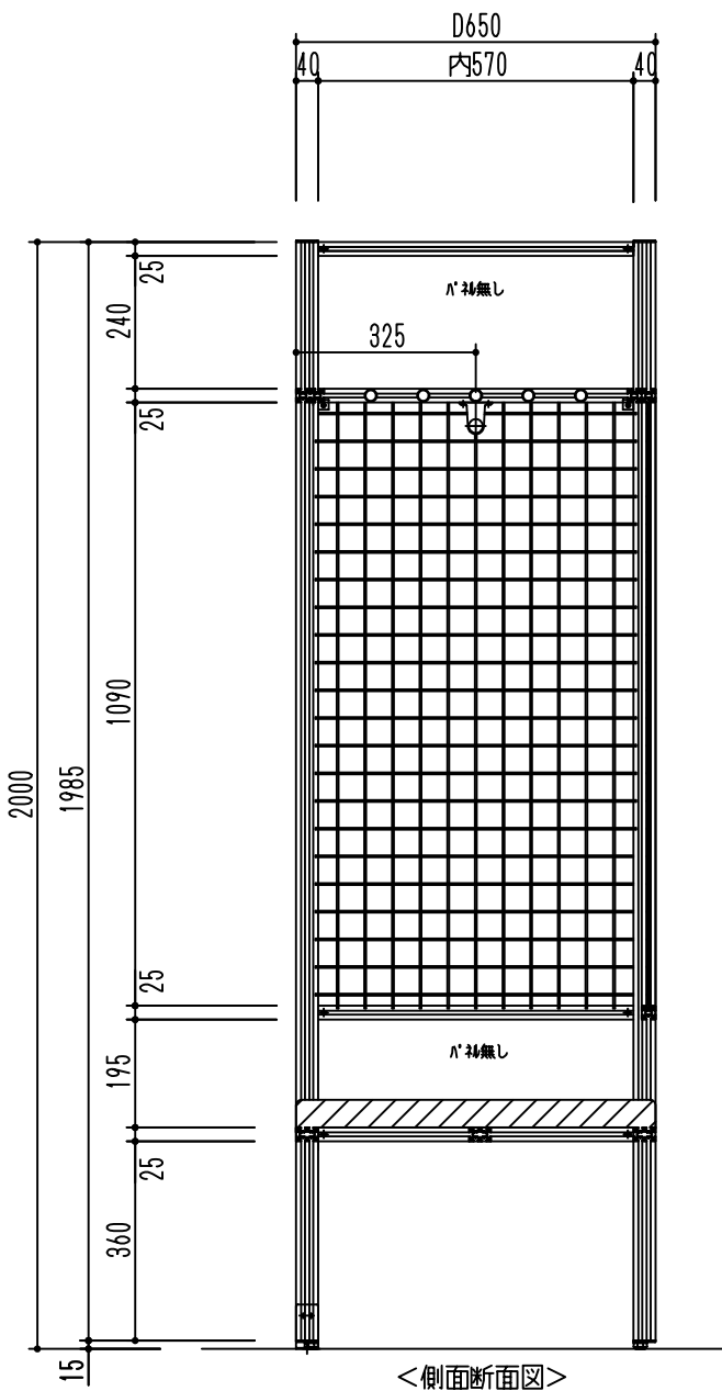
<側面断面図>
