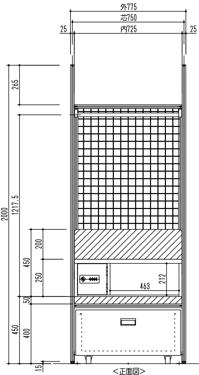
<正面図>
