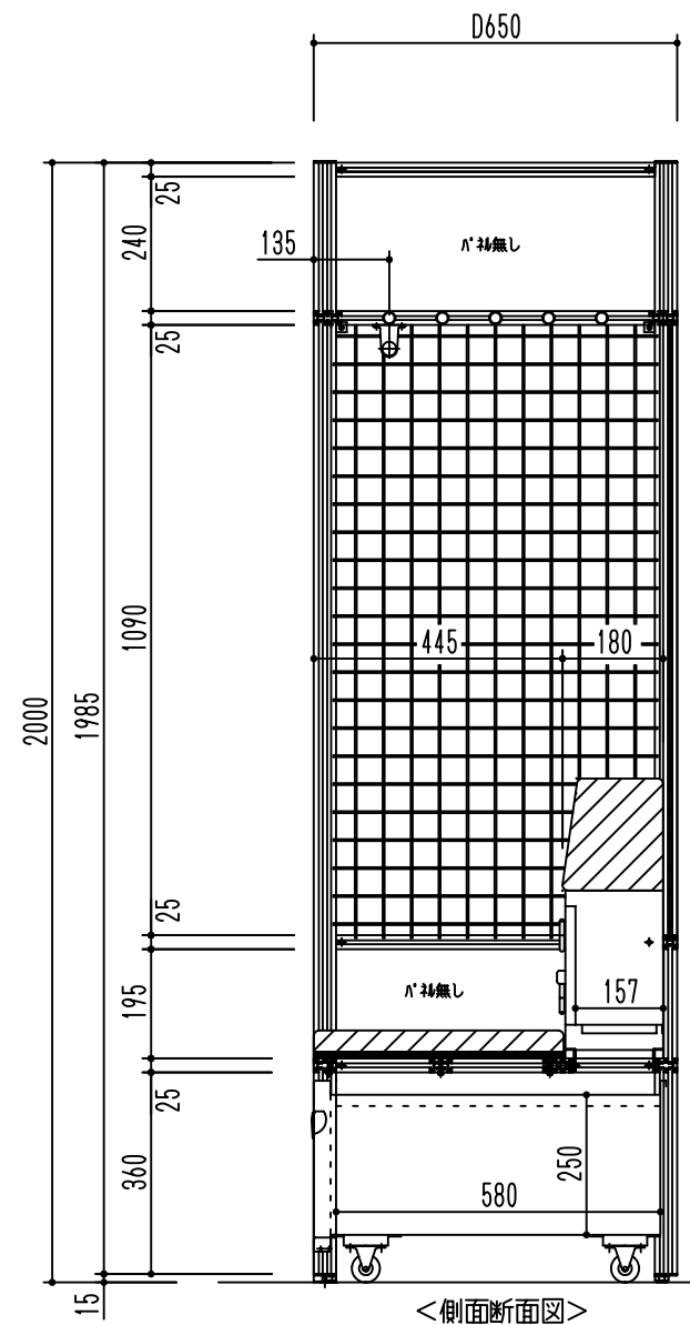
<側面断面図>
