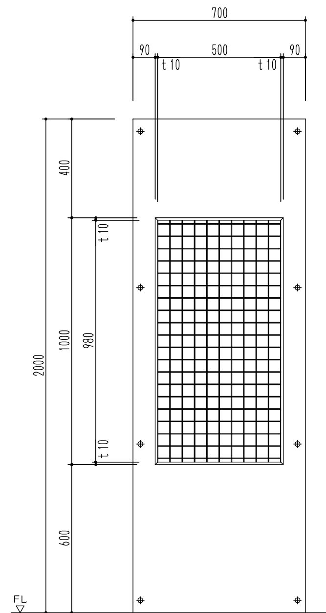
<側面図>
