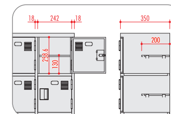
ST4-6 (24人用) H1730×W1058×D350 横中仕切板溶接固定、名札差プレス加工、中棚付
