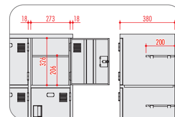
SW3-5 (15人用) H1790×W891×D380 横中仕切板溶接固定、名札差プレス加工、中棚付
