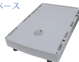
PLE-BS-L ロッカー用ベース(1 列用) H55(65) × W308 × D465 再生材プラスチック、アジャスター付
