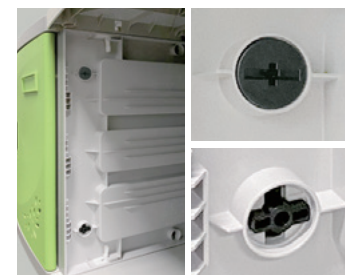
PLE-LRC-L ロッカー用左右連結パーツ PLE-LRC-S シューズケース用左右連結パーツ
