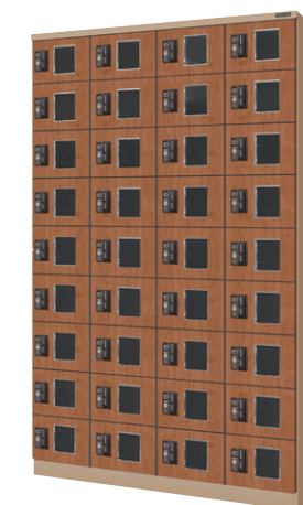
YMP4-9 (4列9段 36人用) H1800×W1100×D350 扉寸H185.33×W267 扉：ポリカーボネート窓付、木目シート貼仕上 ※ピンヒンジ仕様
