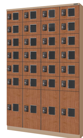
YMP4-7 (4列7段 28人用) H1800×W1100×D350 上段：扉寸H185.33×W267 最下段：扉寸H564×W267 扉：ポリカーボネート窓付、木目シート貼仕上 ※ピンヒンジ仕様
